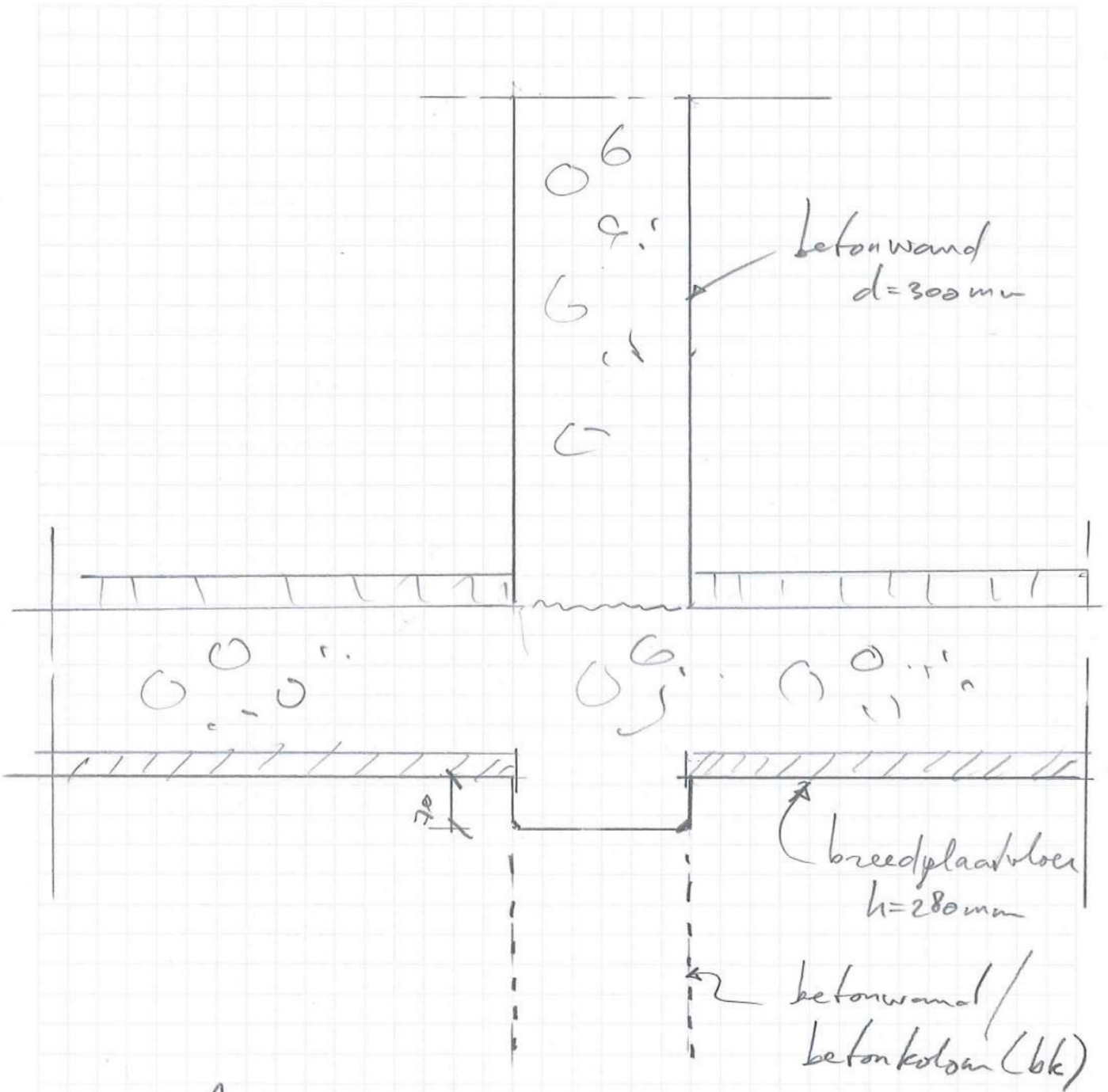
Detail wand ligger (WL)
